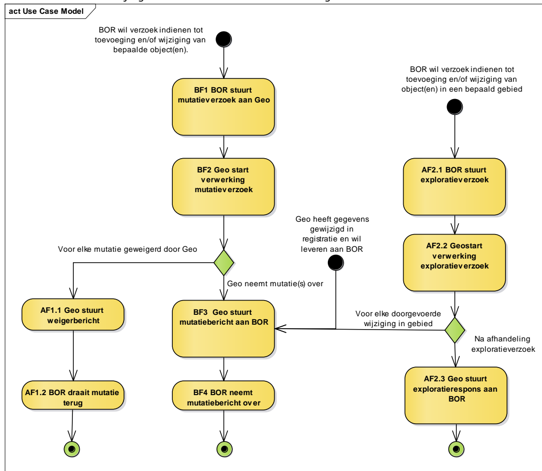
Figuur B1-1 Activiteitendiagram Geo-BOR berichtenverkeer
